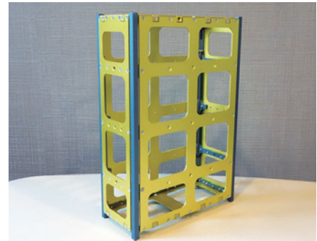
人工衛星の構体設計開発
